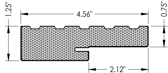
1 JAMB
